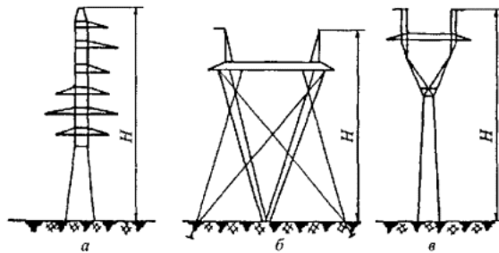
Рис. П8.5. Схемы металлических опор 110 и 330 кВ:
