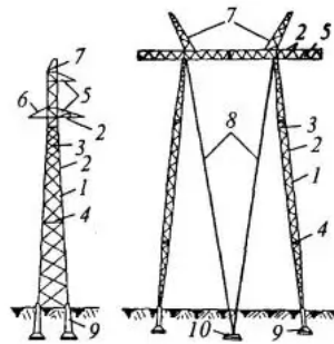
Рис. П8.3. Детали металлических опор и их элементы:
