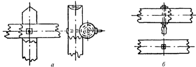
Рис. 5.1. Устройство шунтирующего бандажа:
