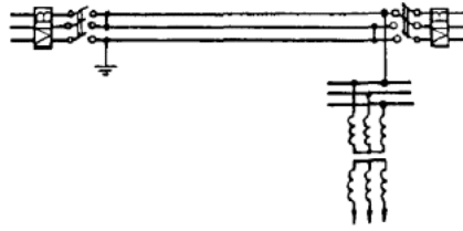
Рис. 5.4. Схема плавки гололеда с последовательным соединением проводов фаз линии при последовательном соединении проводов всех фаз - по схеме «змейка» (рис. 5.4); встречного включения фаз трансформаторов (рис. 5.5);
