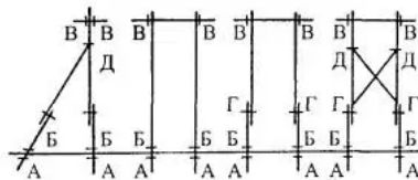
Рис. 3.1. Опасные сечения деревянных опор:
