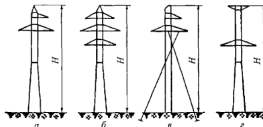
Рис. П8.4. Схемы металлических опор 35-330 кВ:
