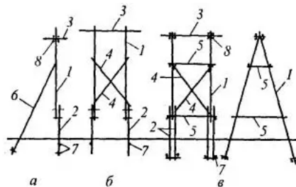
Рис. П8.7. Схемы деревянных опор ВЛ 35-220 кВ и их детали:
