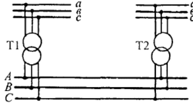
Рис. 5.5. Схема плавки гололеда с встречным включением фаз трансформаторов перераспределения нагрузок в сети путем повышения токовой нагрузки обогреваемой линии; наложения дополнительных токов на рабочий ток обогреваемой ВЛ. 5.8.8. Длины ВЛ, на которых может быть выполнена плавка гололеда на проводах способом трехфазного короткого замыкания при различных напряжениях плавки, приведены в табл. 5.3. 5.8.9. Плавка гололеда на грозозащитных тросах может производиться токами короткого замыкания, искусственно создаваемого на ВЛ, или встречным включением фаз трансформаторов. При плавке гололеда на грозозащитных тросах в зависимости от напряжения плавки трос должен быть изолирован на опорах ВЛ: с помощью одного изолятора при напряжении плавки 3-20 кВ, двух изоляторов - 35 кВ, четырех изоляторов - 110 кВ.
