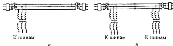
Рис. 5.3. Схемы плавки гололеда с замыканием трех фаз:
