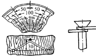
Рис. 5.2. Закрепление шунтирующего бандажа гвоздями
