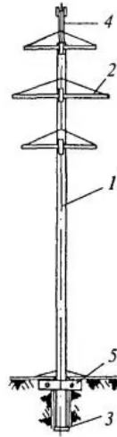
Рис. П8.1. Детали железобетонной свободностоящей опоры:
