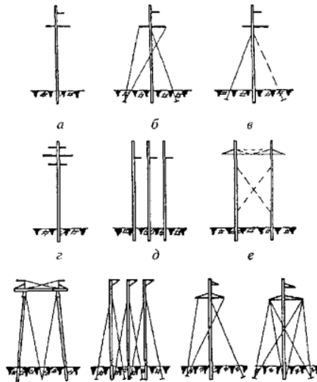
Рис. П8.2. Схемы железобетонных опор 35 - 500 кВ:
