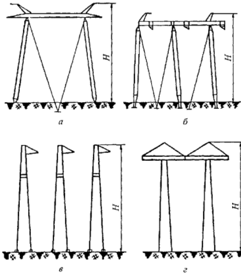
Рис. П8.6. Схемы металлических опор 500-750 кВ:
